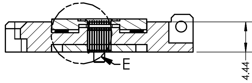
SECTION D-D SCALE 3 : 1
